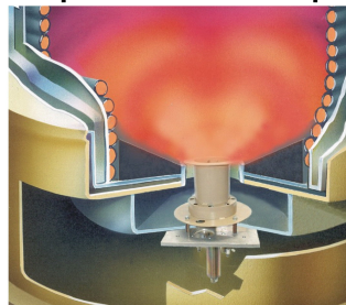
Горивна камера
