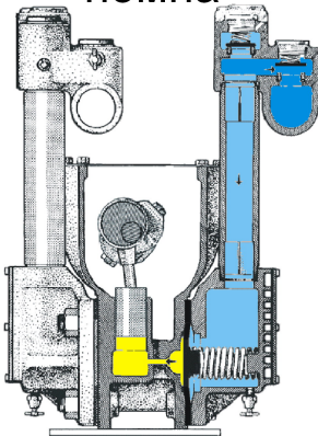
Clayton помпа
